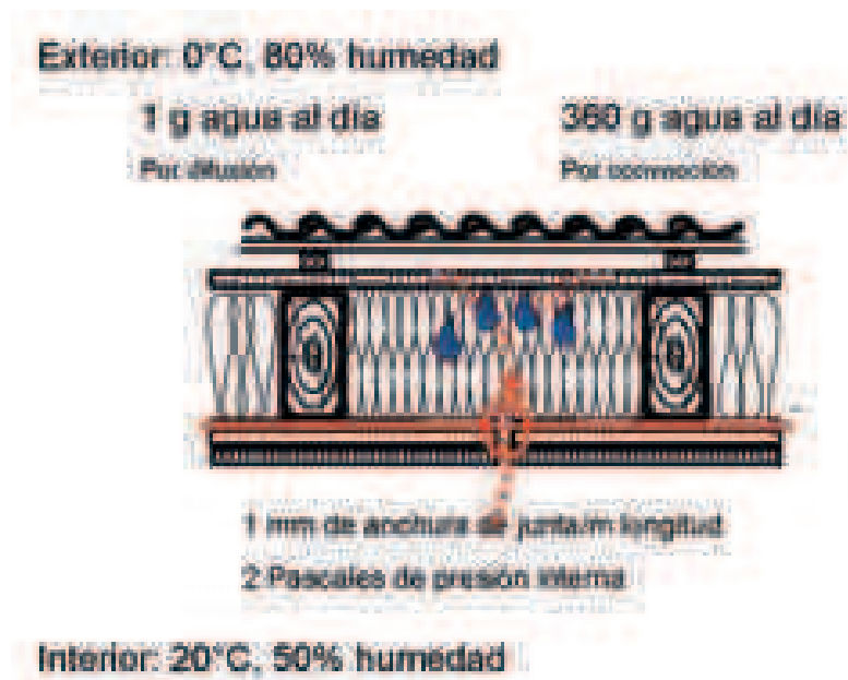
Figura 1. Cubierta de madera. Paso de agua. Fuente: Blowerdoor GmbH.
