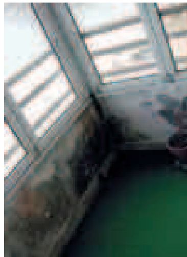
Fotografía 2. Efectos de condensación en puentes térmicos. Fuente: Javier Crespo.
