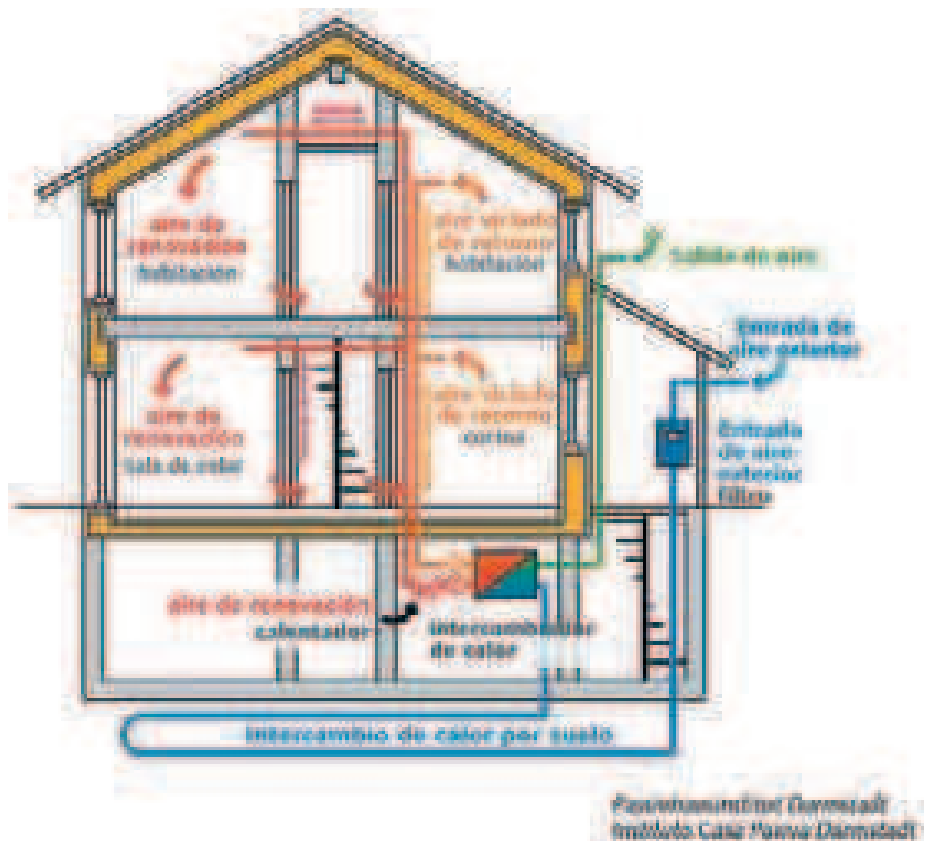
Figura 1. Croquis esquemático de la eficiencia en la ventilación Passivhaus. Fuente: PHI. Adaptaciones: Construnario.
