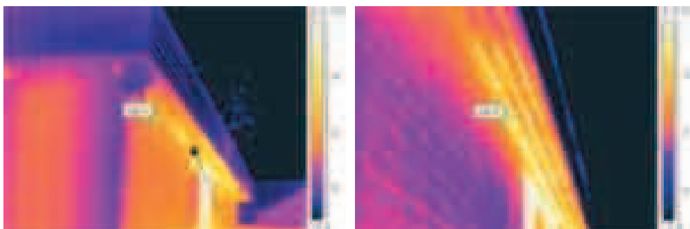
Fotografía 10 y 11. (Izq.). Termograma a presión normal. (Dcha.). Termograma + Presurización.
