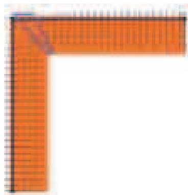
Figura 2. Líneas de flujo de calor en una esquina saliente con la misma solución constructiva que en el caso de la fotografía 1. Puede apreciarse cómo el flujo sufre una desviación respecto de la dirección perpendicular al cerramiento cuando nos acercamos a la esquina.
