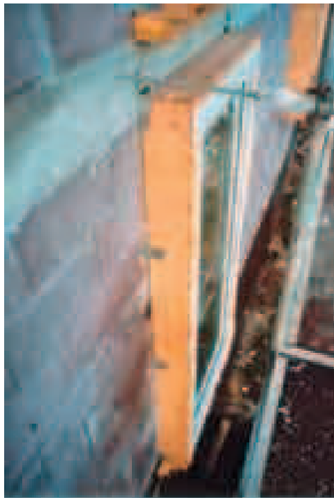
Fotografía 2. Imagen de comprobaciones en obra de la posición de la ventana en el plano del aislamiento térmico.
