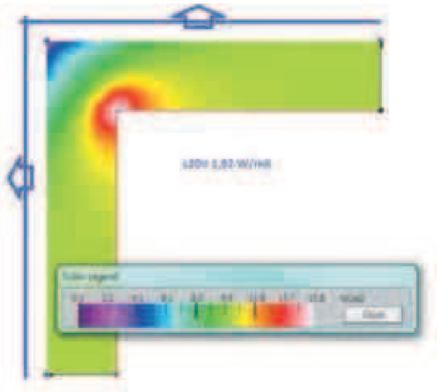
Figura 4. Valores del flujo de calor en los distintos puntos del cerramiento. En azul, cálculo realizado por el software del flujo total de calor por K y m lineal de PT. Fuente: Elaboración propia.
