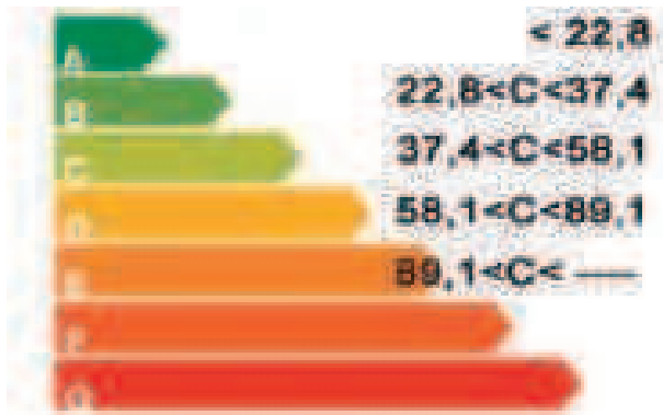
Figura 2. Valores límite entre clases según CTE para la provincia de Lleida. Fuente: normativa CTE: Documento reconocido de las Condiciones para la Aceptación de Programas Alternativos.
