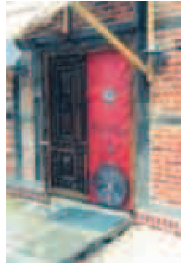
Fotografías 3 y 4. (izq.) Test BlowerDoor en vivienda unifamiliar de nueva construcción. (dcha.) Test BlowerDoor en rehabilitación de edificio con estructura de madera.
